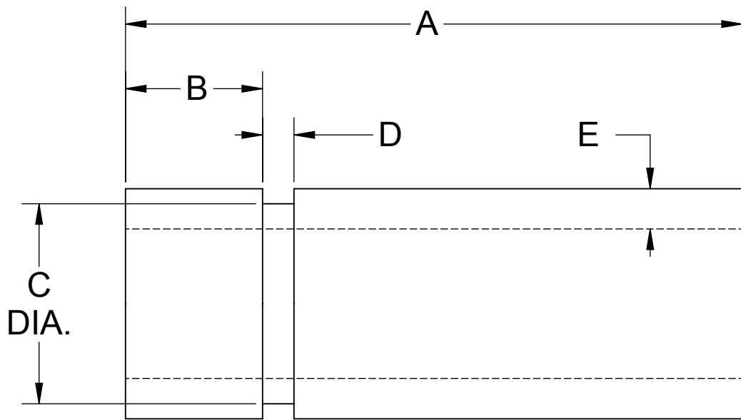
RING GROOVE DIMENSIONS
